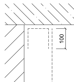
Schéma prekrývania výstužnej mriežky
