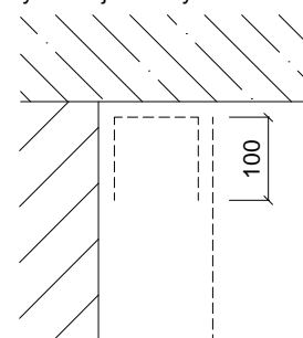
Schéma prekrývania výstužnej mriežky
