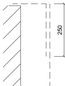
Schéma prekrývania výstužnej mriežky
